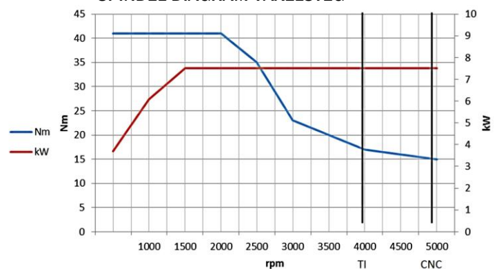
SPINDEL DIAGRAM VÄXELSTEG
